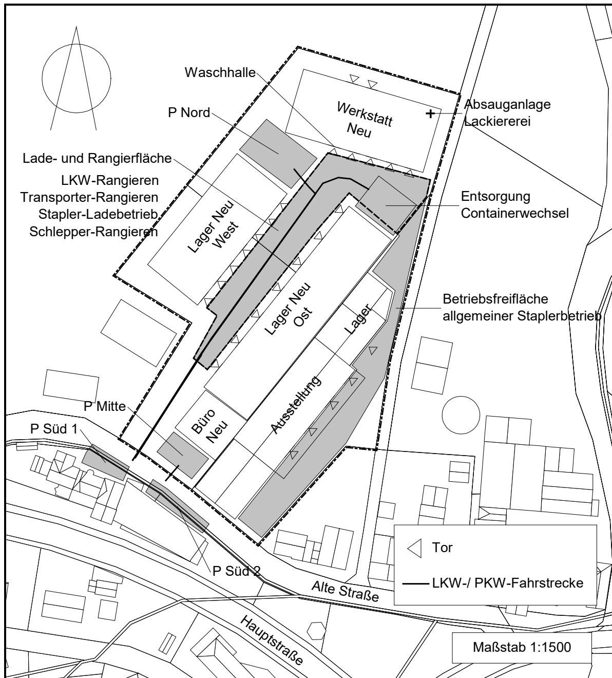
Abbildung 3: Lageplan Emissionsquellen
