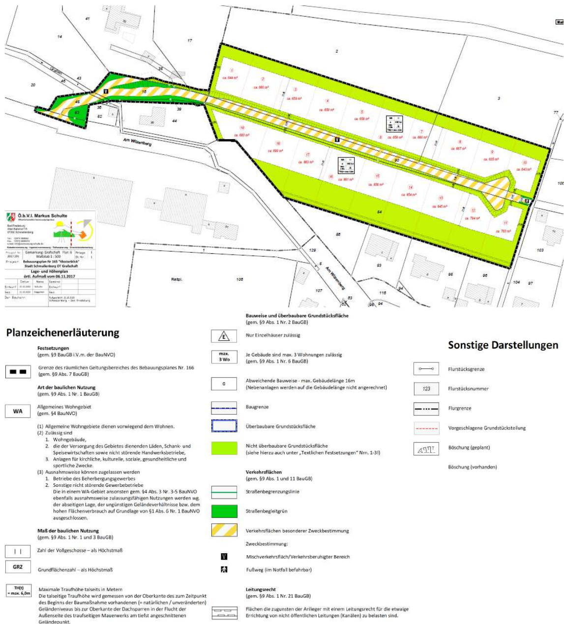
Abb. 2 Auszug aus der Planzeichnung des Bebauungsplanes Nr. 165 „Klosterblick“ (SCHULTE 2020B).
