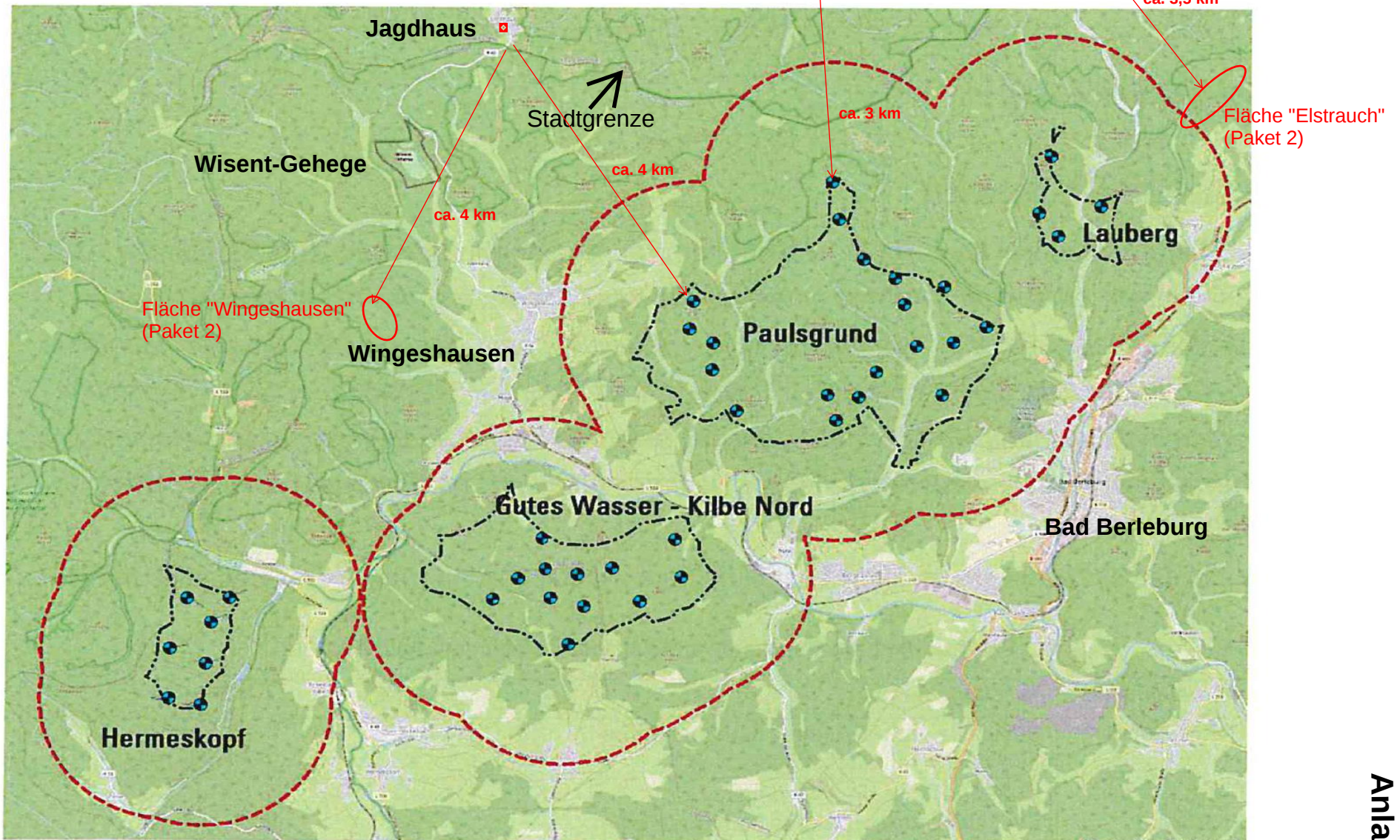
Abb. 6 Übersicht der Untersuchungsgebiete mit 10-fachem Rotorradius = 1.700 m (rote Linie), Potenzialflächen (schwarze Linien) und geplanten WEA (blaue Markierungen)
