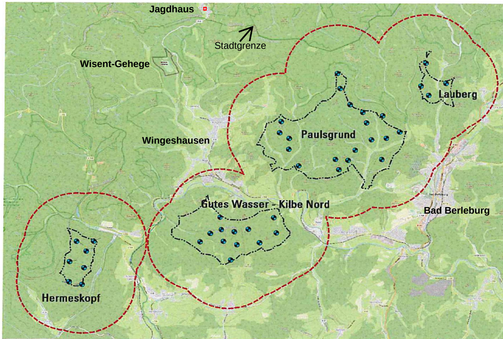
Abb. 6 Übersicht der Untersuchungsgebiete mit 10-fachem Rotorradius = 1.700 m (rote Linie), Potenzialflächen (schwarze Linien) und geplanten WEA (blaue Markierungen)
