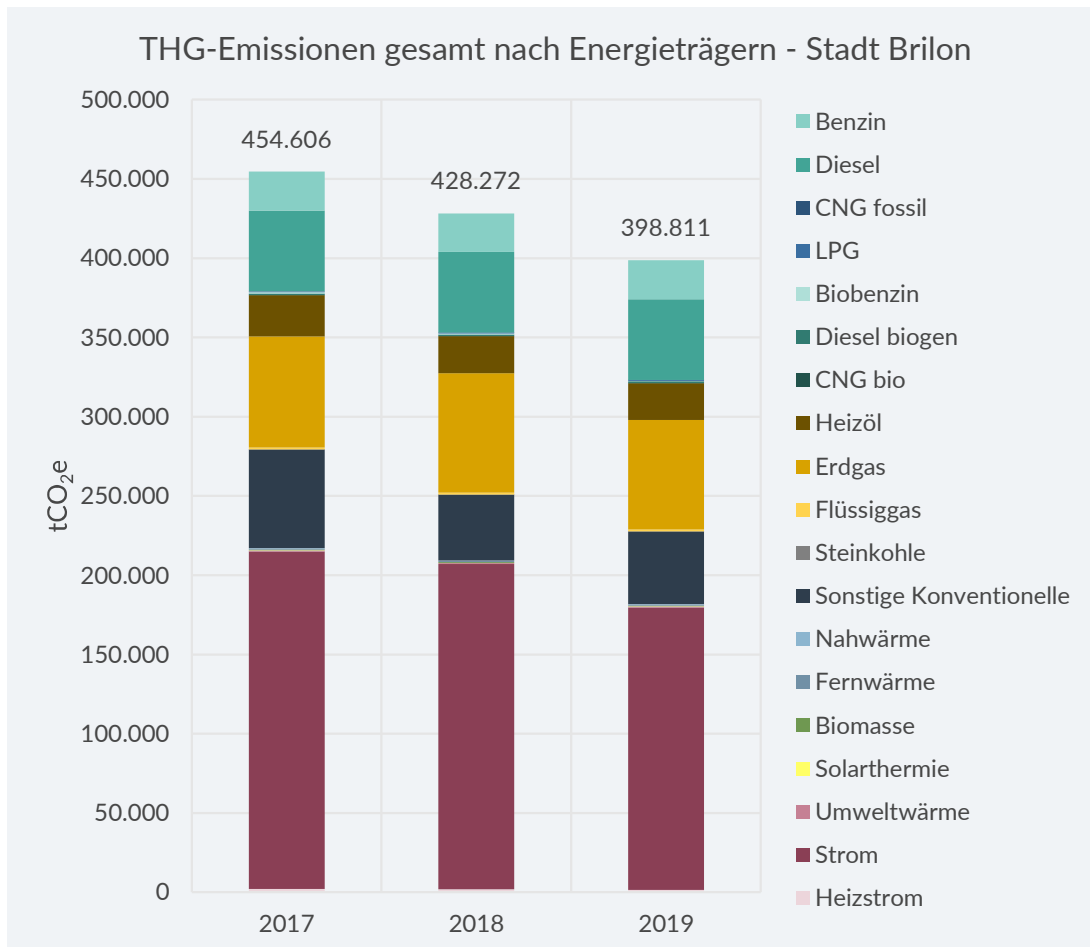
Abbildung 7-28: THG-Emissionen der Stadt Brilon nach Energieträgern
