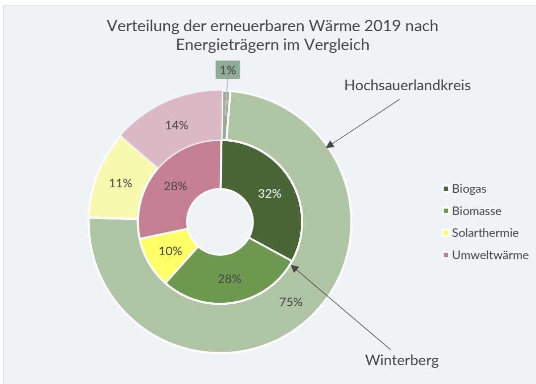
Abbildung 7-196: Vergleich Verteilung der erneuerbaren Wärme nach Energieträgern in der Stadt Winterberg und dem HSK für das Jahr 2019
