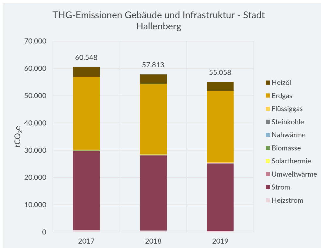
Abbildung 7-64: THG-Emissionen der Gebäude und Infrastruktur nach Energieträgern der Stadt Hallenberg
