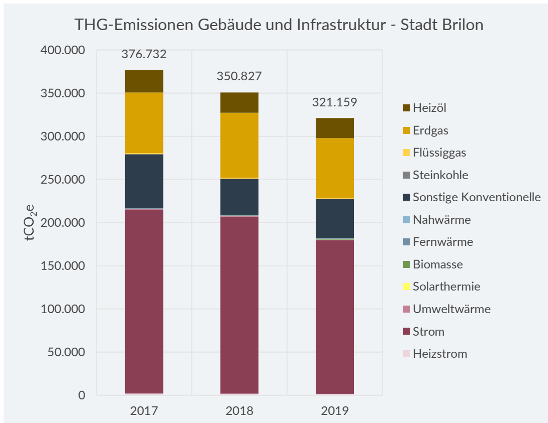
Abbildung 7-29: THG-Emissionen der Gebäude und Infrastruktur nach Energieträgern der Stadt Brilon
