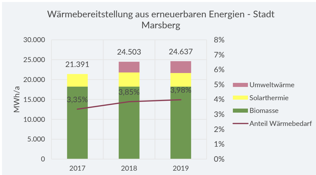
Abbildung 7-87: Wärmebereitstellung aus erneuerbaren Energien nach Energieträgern in der Stadt Marsberg Im Bilanzjahr 2019 entfielen die Anteile an der erneuerbaren Wärmebereitstellung auf Biomasse (74 %), Solarthermie (14 %) und Umweltwärme (12 %).
