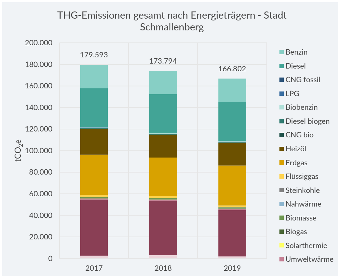
Abbildung 7-153: THG-Emissionen der Stadt Schmallingenberg nach Energieträgern
