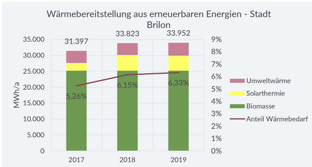
Abbildung 7-34: Wärmebereitstellung aus erneuerbaren Energien nach Energieträgern in der Stadt Brilon
