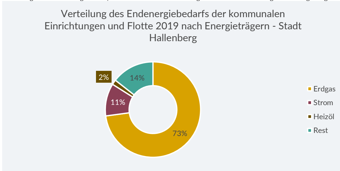
Abbildung 7-60: Anteil der Energieträger am Endenergiebedarf der kommunalen Einrichtungen der Stadt Hallenberg
