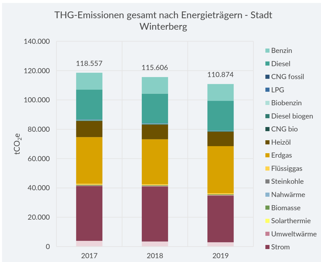
Abbildung 7-189: THG-Emissionen der Stadt Winterberg nach Energieträgern
