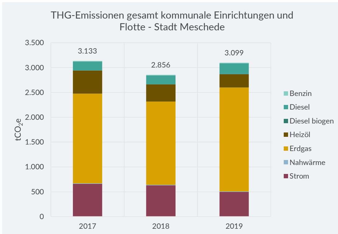
Abbildung 7-119: THG-Emissionen der kommunalen Einrichtungen der Stadt Meschede nach Energieträgern
