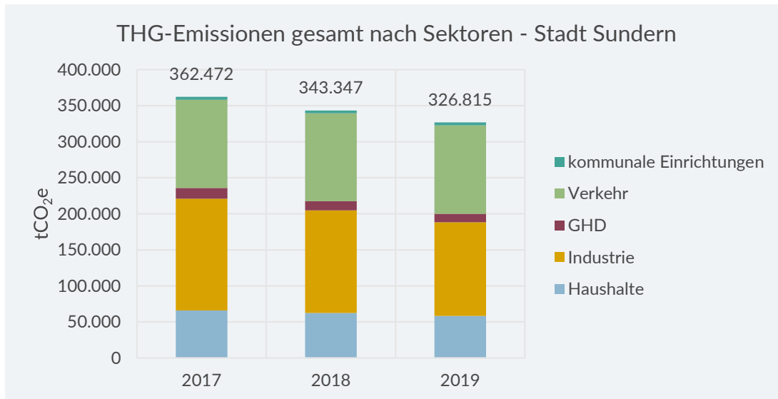
Abbildung 7-169: THG-Emissionen der Stadt Sundern nach Sektoren
