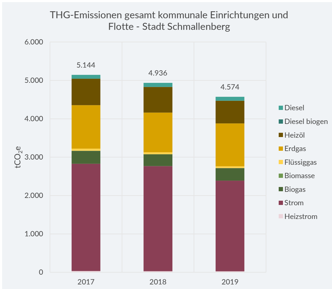
Abbildung 7-155: THG-Emissionen der kommunalen Einrichtungen der Stadt Schmallenberg nach Energieträgern
