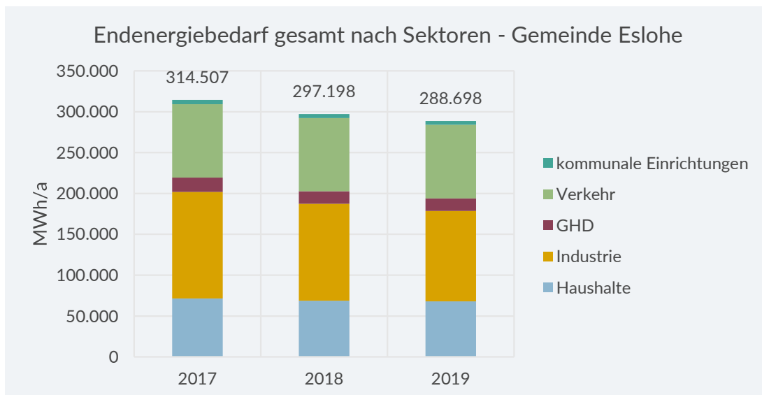
Abbildung 7-38: Endenergiebedarf nach Sektoren der Gemeinde Eslohe
