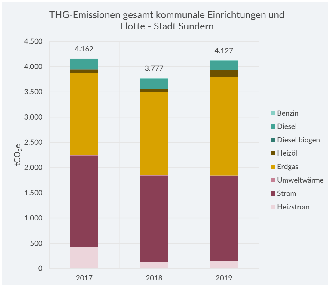
Abbildung 7-173: THG-Emissionen der kommunalen Einrichtungen der Stadt Sundern nach Energieträgern
