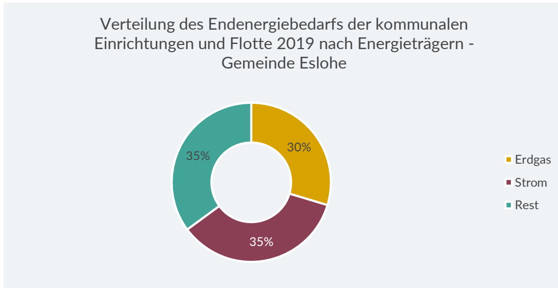
Abbildung 7-43: Anteil der Energieträger am Endenergiebedarf der kommunalen Einrichtungen der Gemeinde Eslohe
