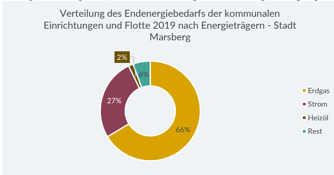
Abbildung 7-78: Anteil der Energieträger am Endenergiebedarf der kommunalen Einrichtungen der Stadt Marsberg
