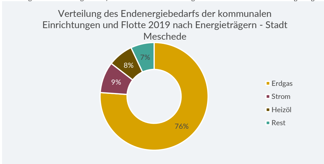
Abbildung 7-114: Anteil der Energieträger am Endenergiebedarf der kommunalen Einrichtungen der Stadt Meschede
