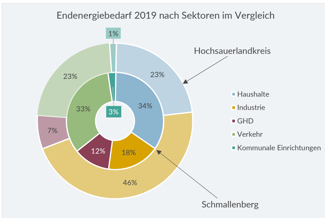
Abbildung 7-146: Vergleich Anteile der Sektoren am Endenergiebedarf der Stadt Schmallingenberg und dem HSK im Jahr 2019
