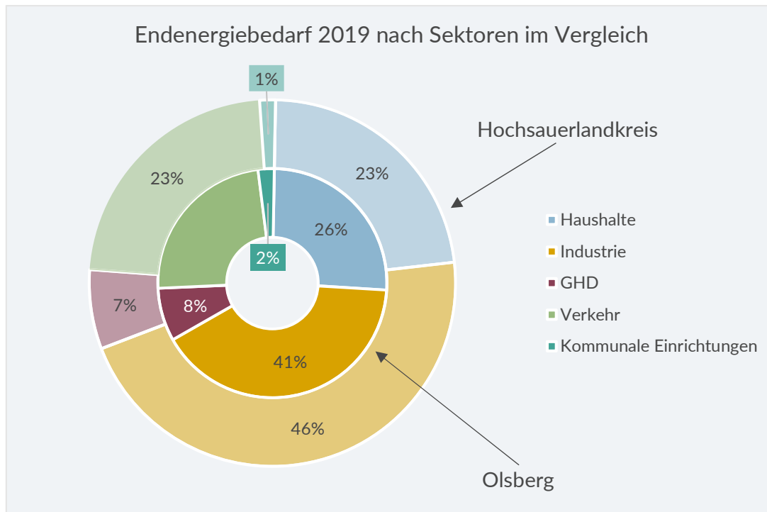
Abbildung 7-128: Vergleich Anteile der Sektoren am Endenergiebedarf der Stadt Olsberg und dem HSK im Jahr 2019
