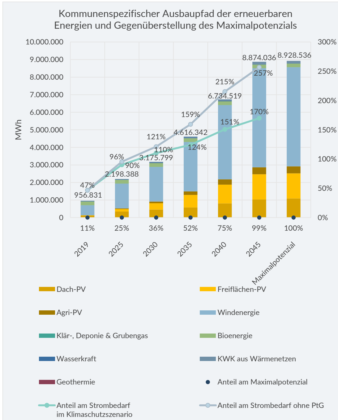
Abbildung 6-10: Kreisspezifischer Ausbaupfad der erneuerbaren Energien und Gegenüberstellung des Maximalpotenzials bis zum Zieljahr 2045 (Eigene Berechnung)
