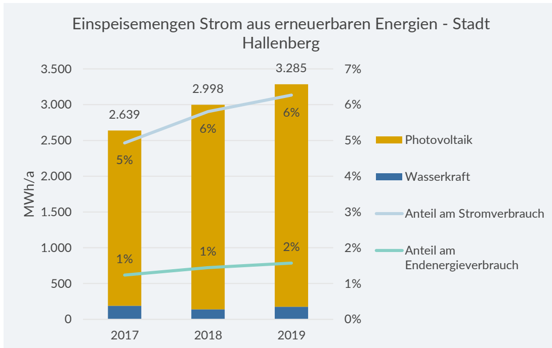
Abbildung 7-66: Strom-Einspeisemengen aus Erneuerbare-Energien-Anlagen der Stadt Hallenberg
