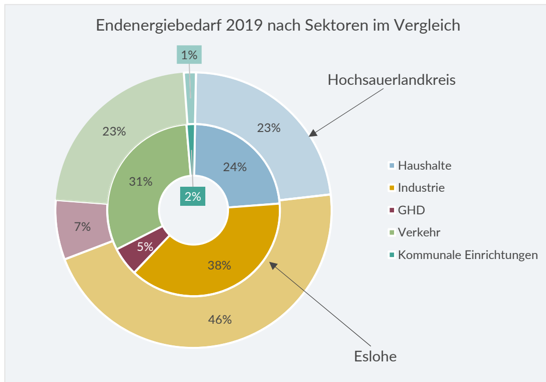
Abbildung 7-39: Vergleich Anteile der Sektoren am Endenergiebedarf der Gemeinde Eslohe und dem HSK in 2019
