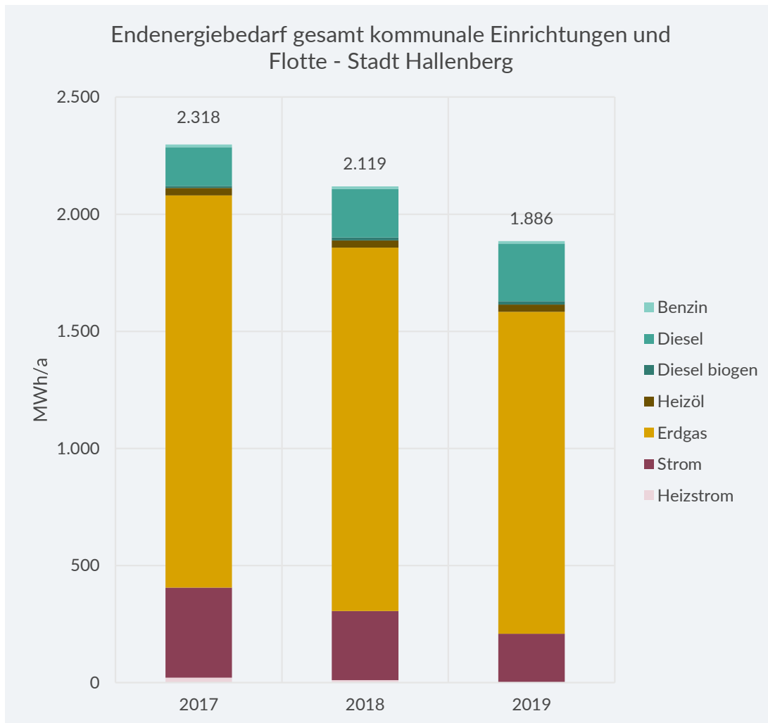
Abbildung 7-59: Endenergiebedarf der kommunalen Einrichtungen der Stadt Hallenberg nach Energieträgern
