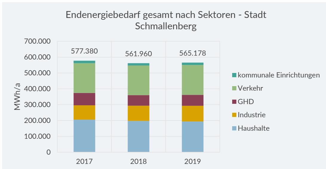
Abbildung 7-145: Endenergiebedarf nach Sektoren der Stadt Schmallingenberg
