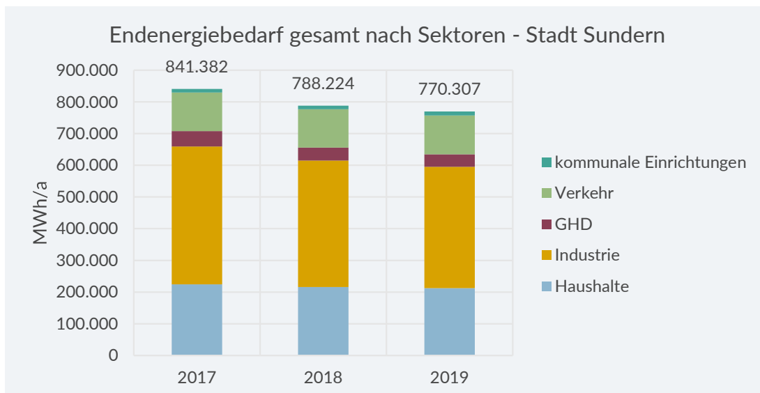
Abbildung 7-163: Endenergiebedarf nach Sektoren der Stadt Sundern
