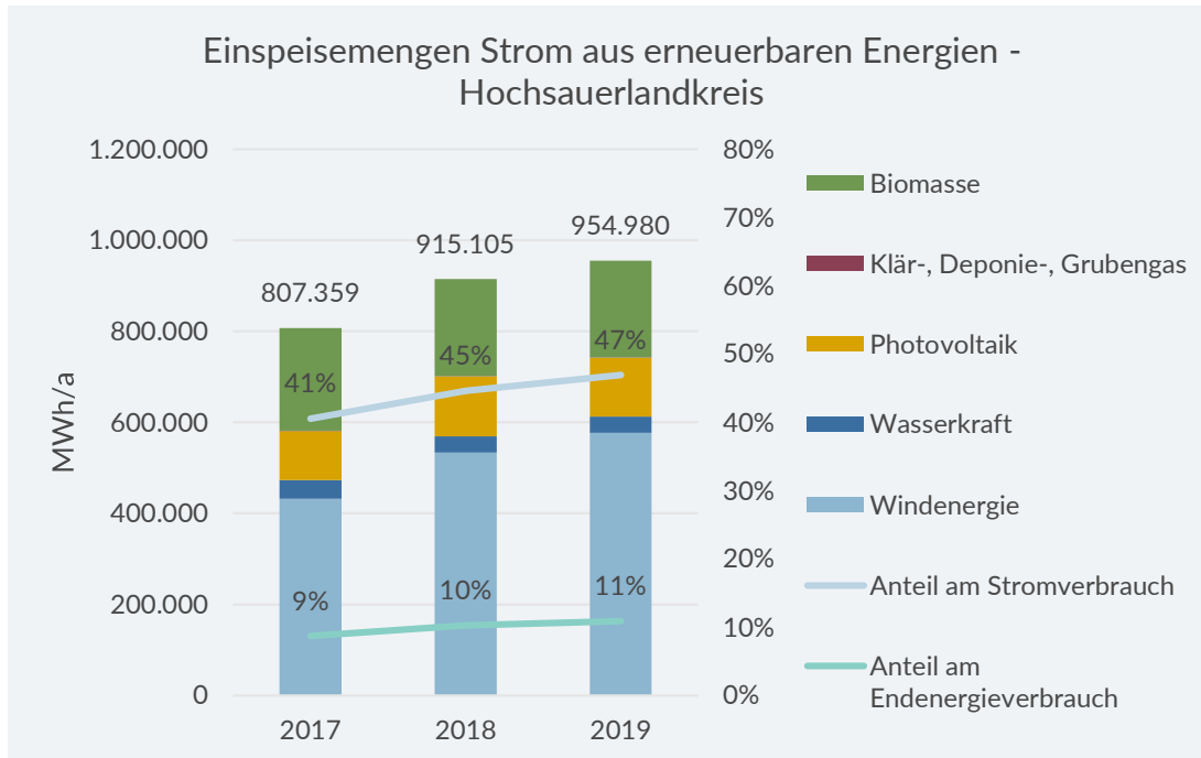
Abbildung 7-158: Strom-Einspeisemengen aus Erneuerbare-Energien-Anlagen im Hochsauerlandkreis
