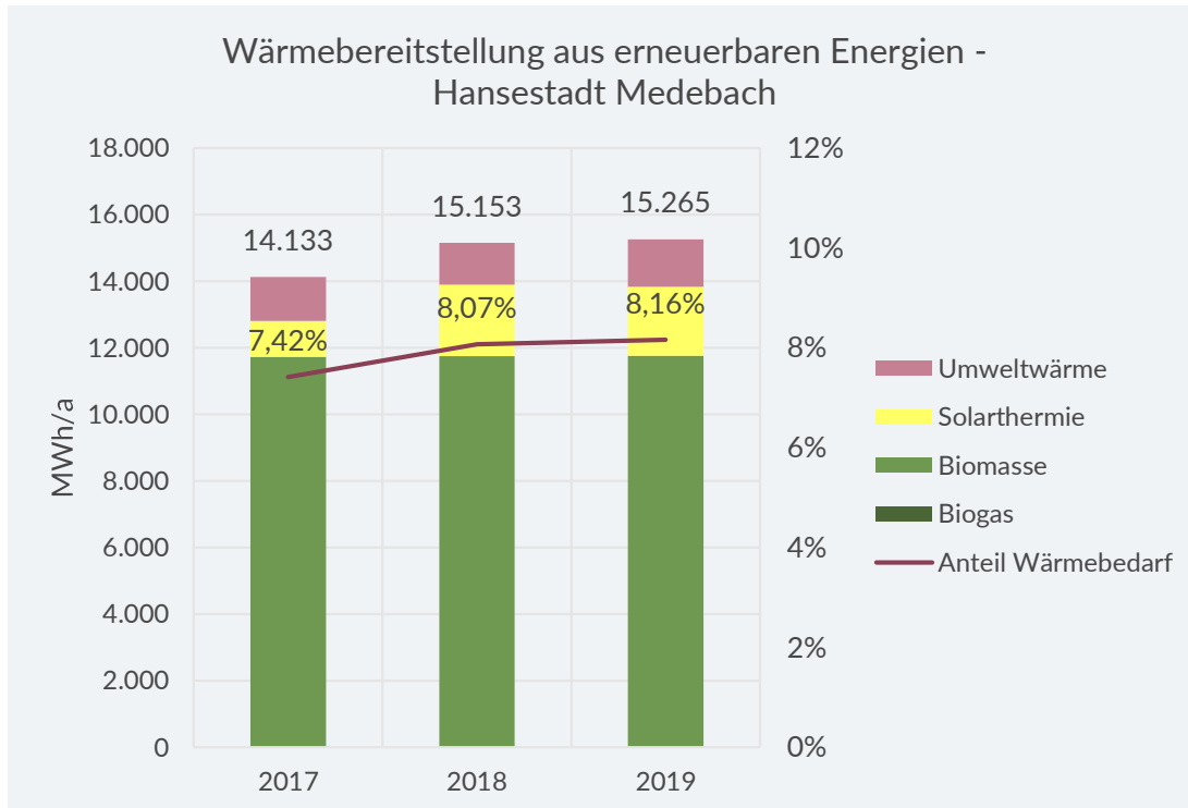
Abbildung 7-105: Wärmebereitstellung aus erneuerbaren Energien nach Energieträgern in der Hansestadt Medebach
