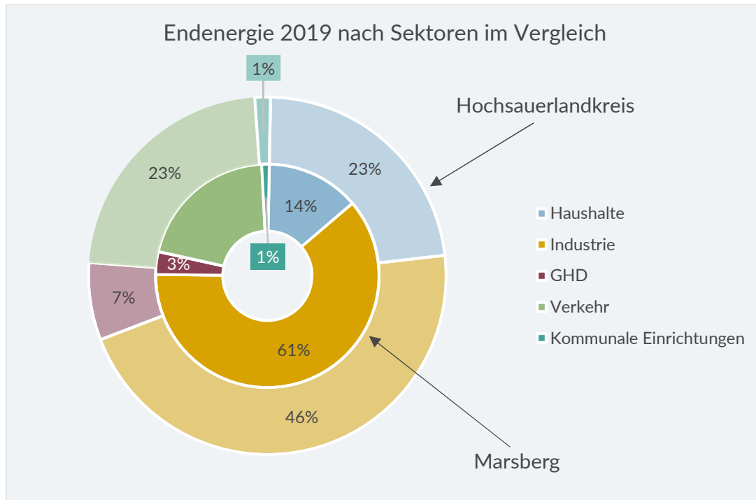
Abbildung 7-74: Vergleich Anteile der Sektoren am Endenergiebedarf der Stadt Marsberg und dem HSK im Jahr 2019
