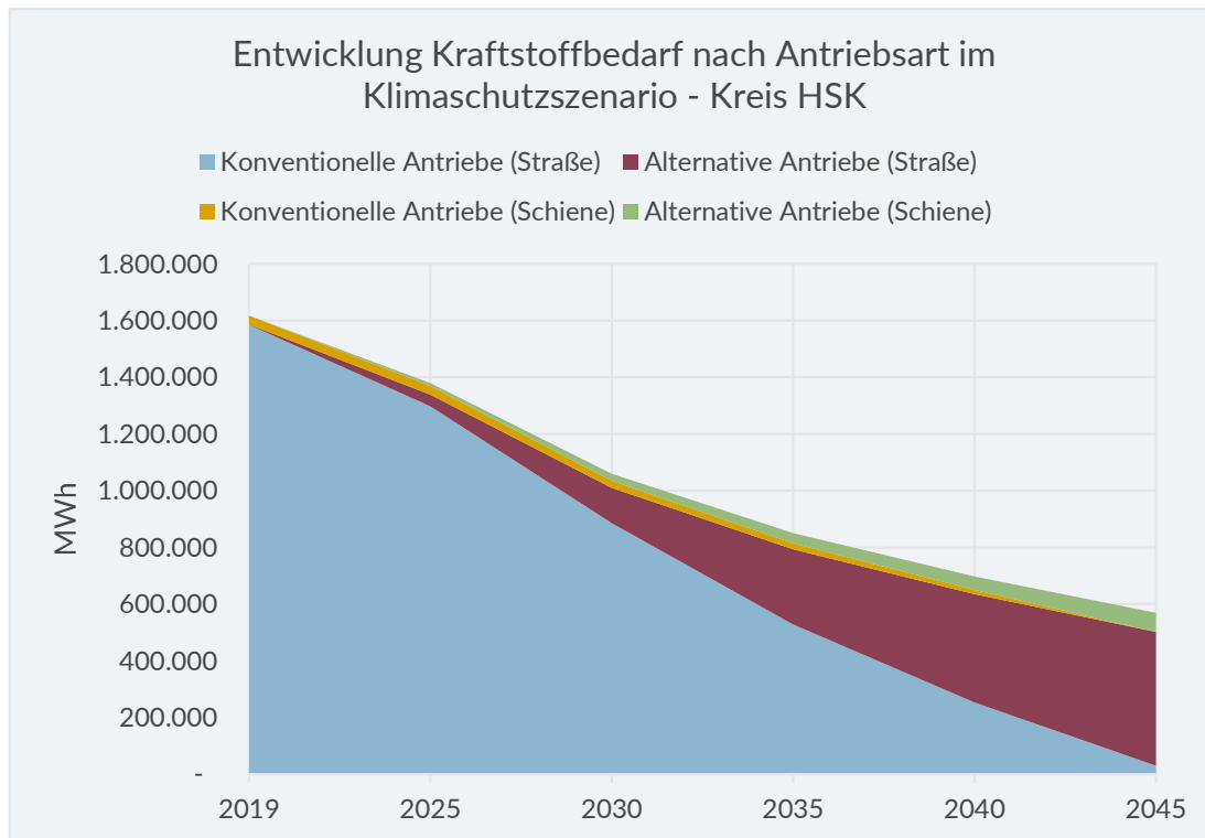
Abbildung 6-6: Zukünftiger Kraftstoffbedarf im Klimaschutzscenario (Eigene Berechnung auf Grundlage witterungskorrigierter Bilanzdaten)
