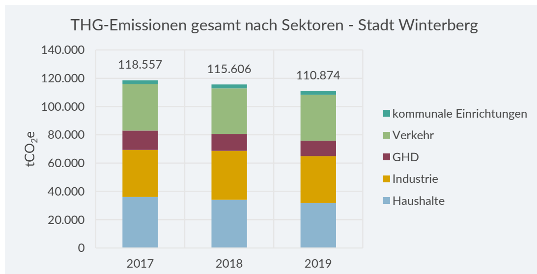
Abbildung 7-187: THG-Emissionen der Stadt Winterberg nach Sektoren
