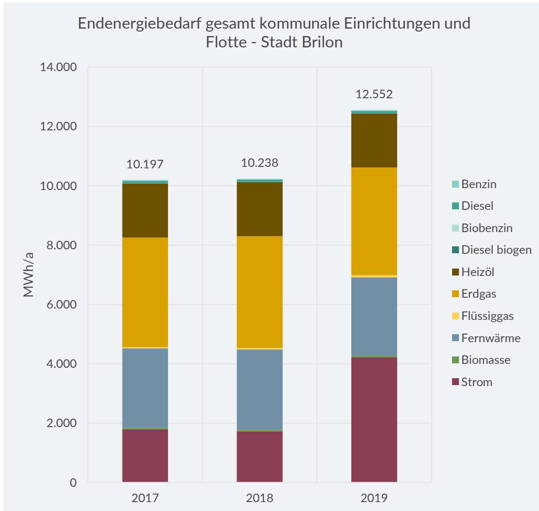
Abbildung 7-24: Endenergiebedarf der kommunalen Einrichtungen der Stadt Brilon nach Energieträgern
