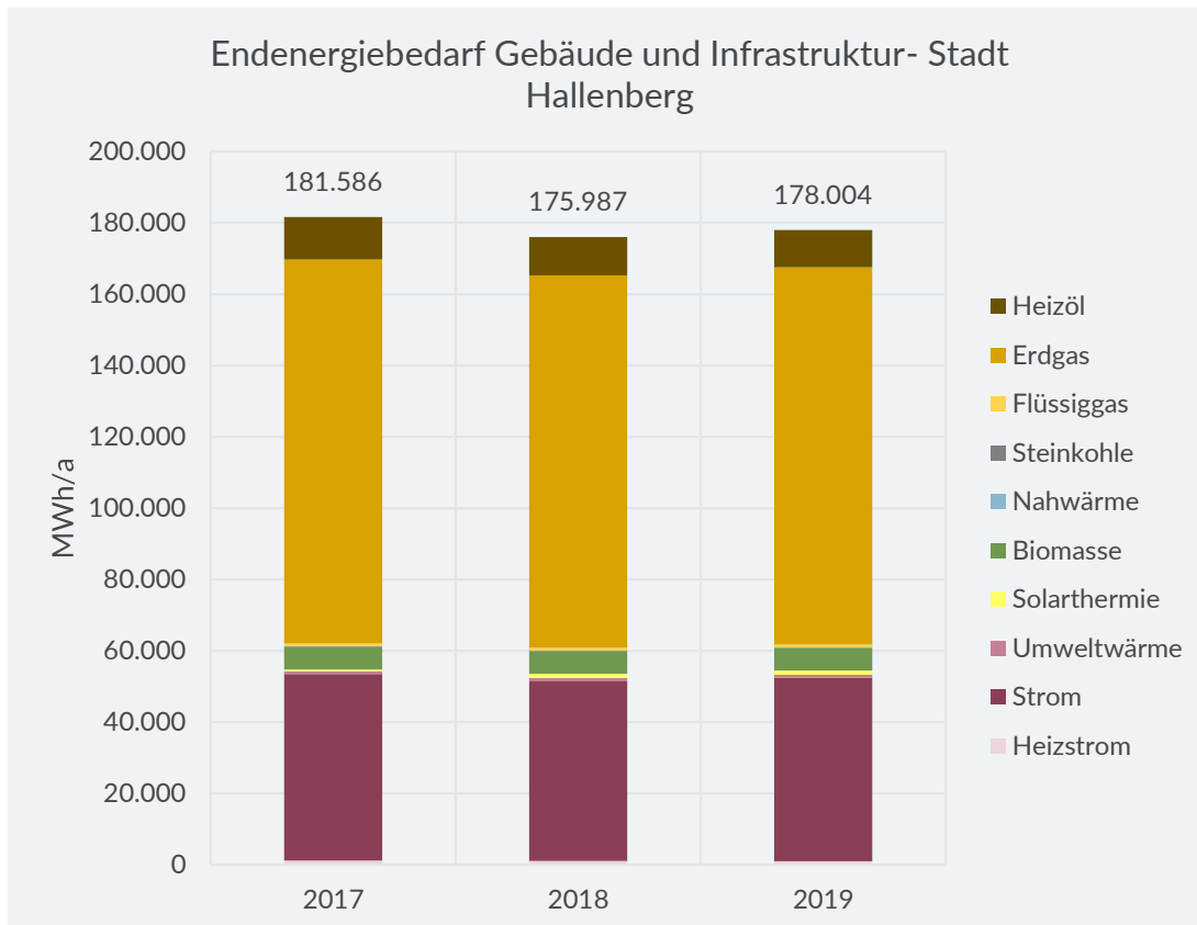
Abbildung 7-58: Endenergiebedarf der Gebäude und Infrastruktur nach Energieträgern der Stadt Hallenberg
