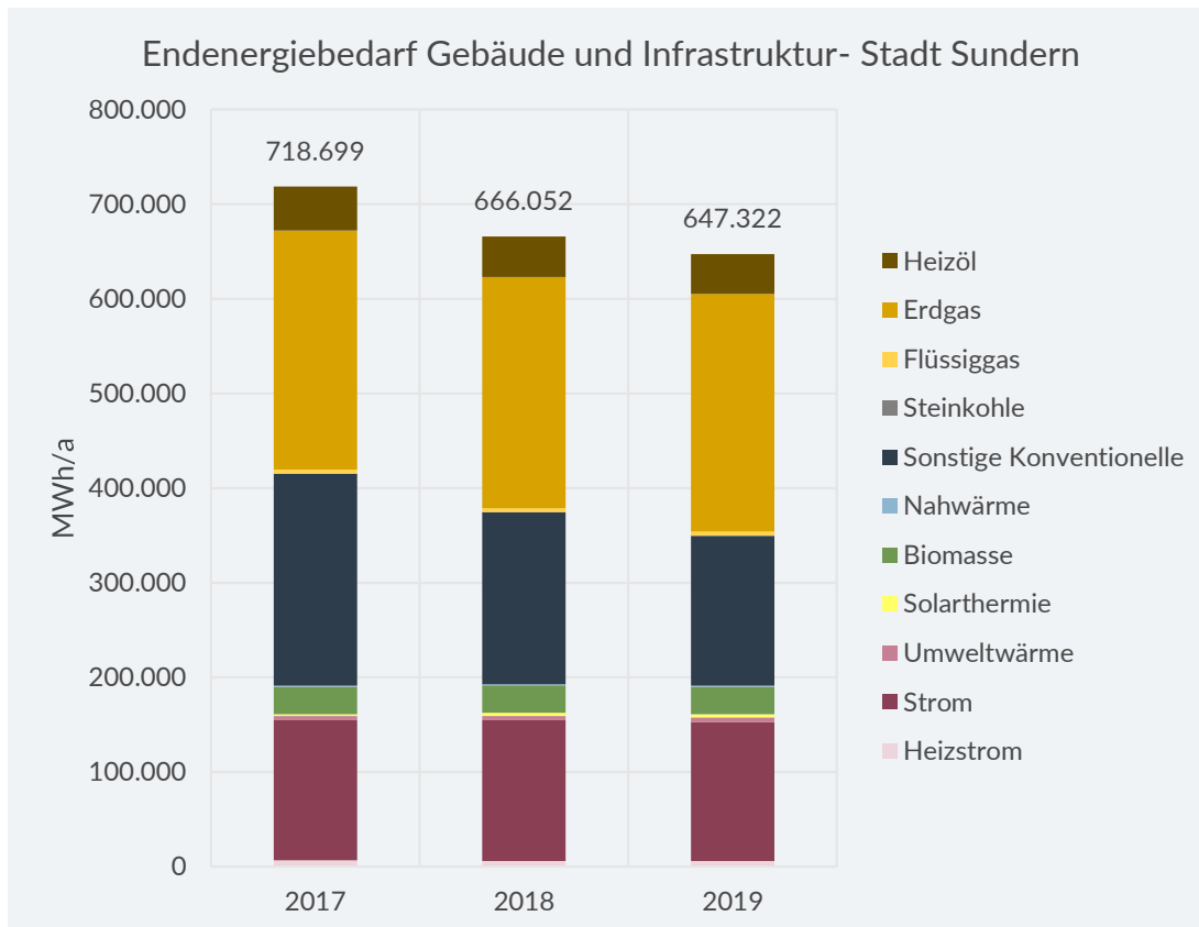
Abbildung 7-166: Endenergiebedarf der Gebäude und Infrastruktur nach Energieträgern der Stadt Sundern
