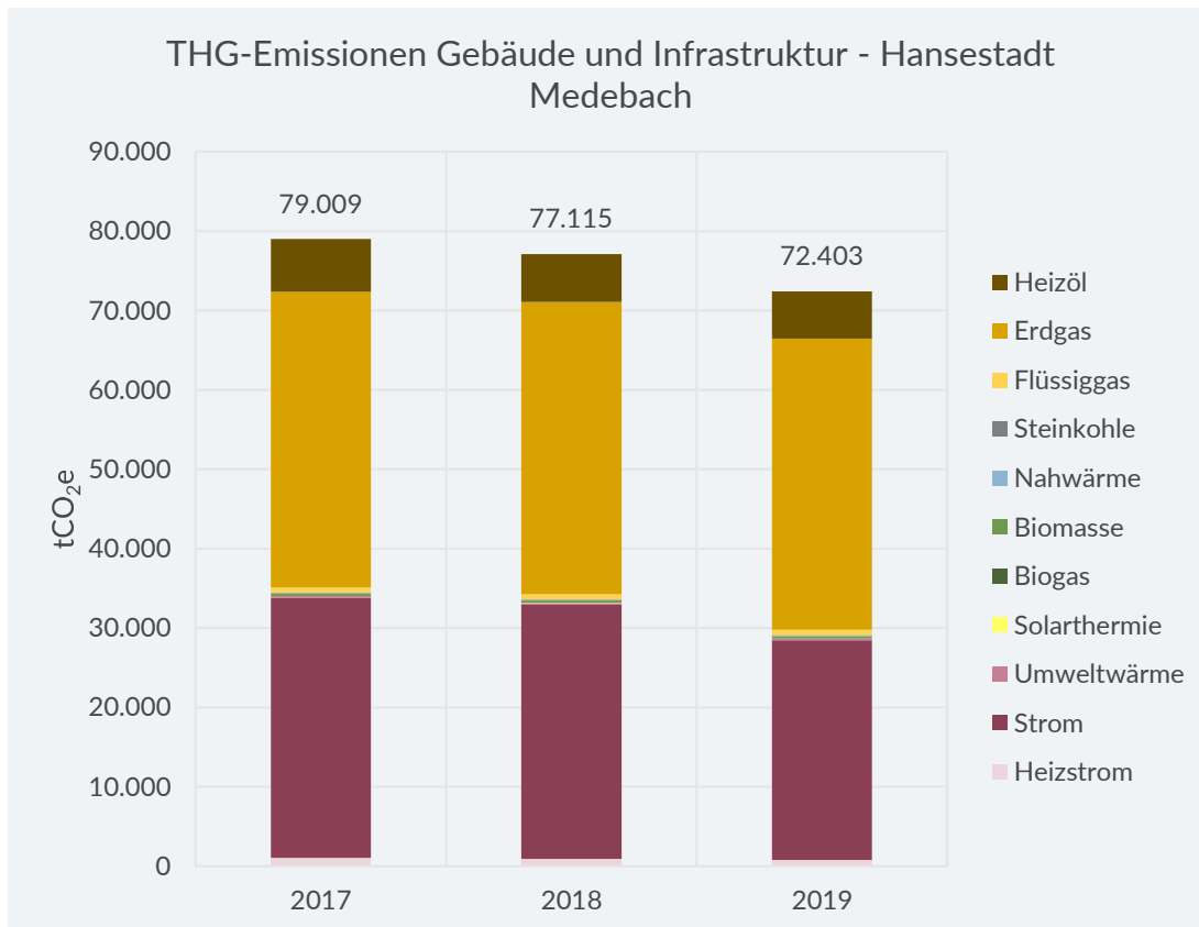
Abbildung 7-100: THG-Emissionen der Gebäude und Infrastruktur nach Energieträgern der Hansestadt Medebach
