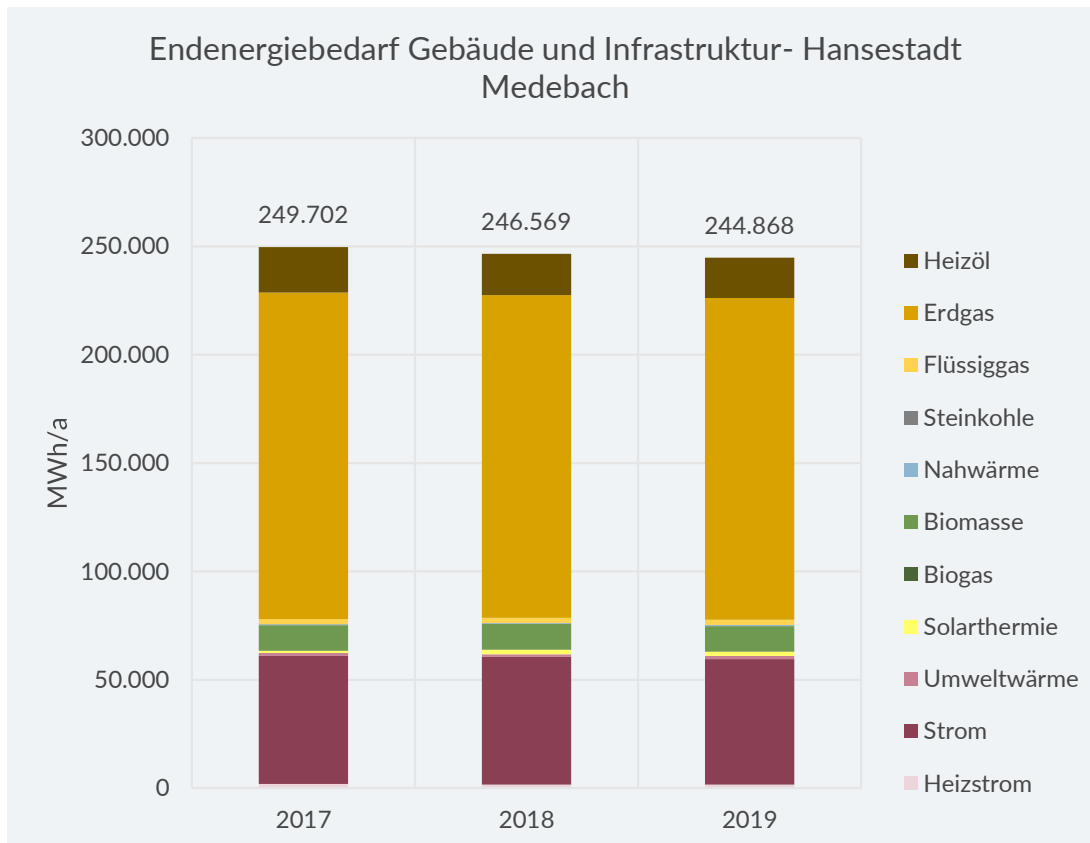
Abbildung 7-94: Endenergiebedarf der Gebäude und Infrastruktur nach Energieträgern der Stadt Medebach
