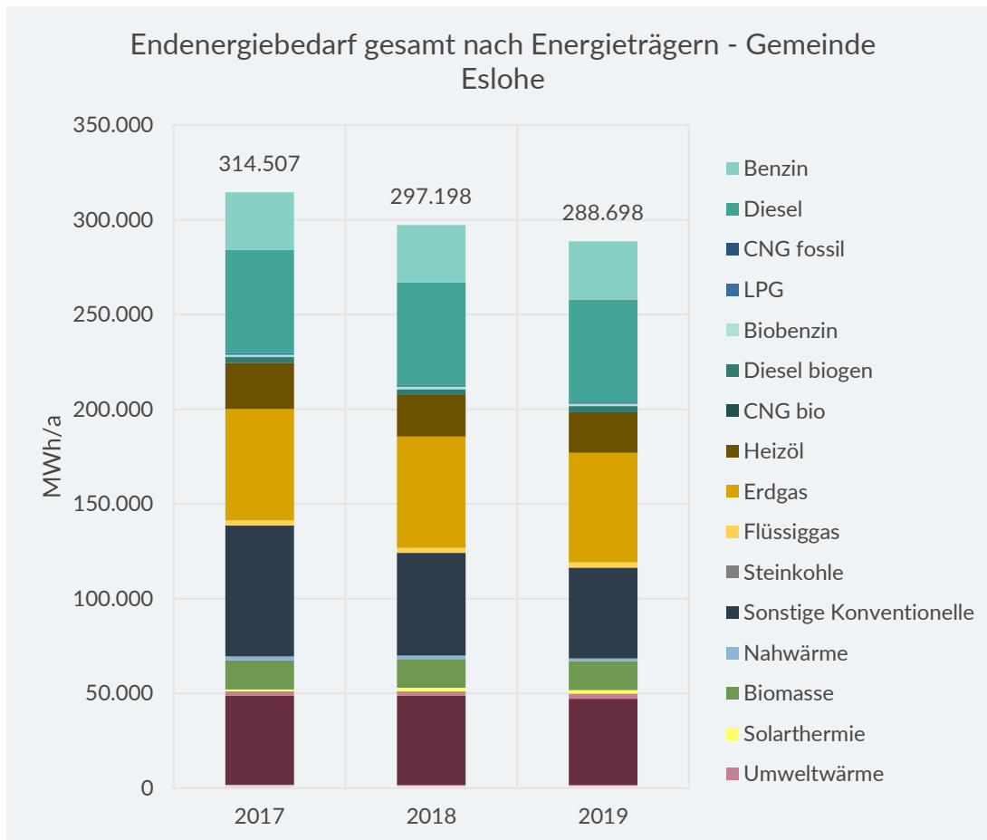
Abbildung 7-40: Endenergiebedarf der Gemeinde Eslohe nach Energieträgern
